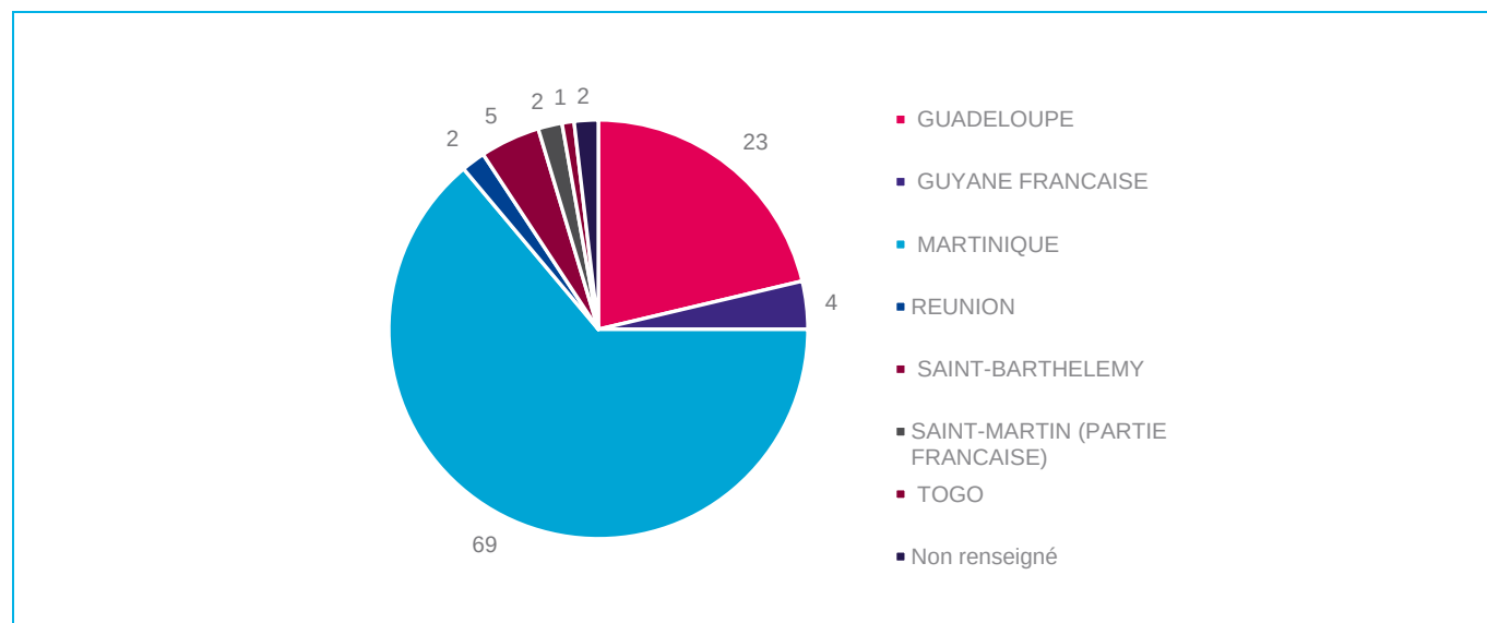
Figure 2 – Répartition des régions d'importation des cas importés confirmés de dengue, région ARA, saison 2020 (n=108)
